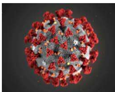
Omicron
